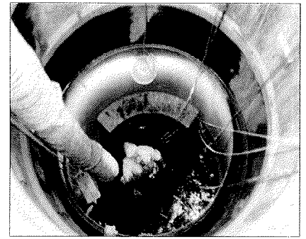
Bild 5: Arbeiten auf der Deponiesohle unter Vollschutz
