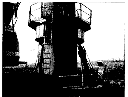
Bild 7: Rohrzieheinrichtung
