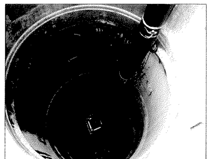
Bild 3: Blick in den Schacht während des Rohreinzuges
