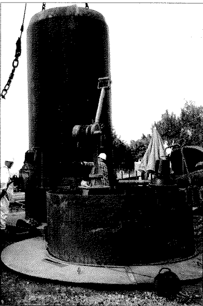
Bild 4: Tunnelpresse vor dem Einsetzen
