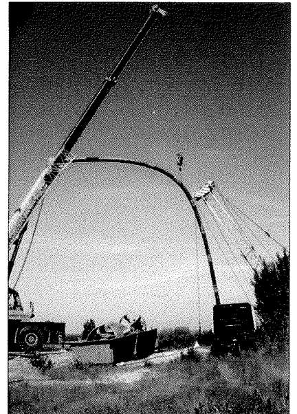
Bild 6: Einzug der neuen PE-HD Leitung
