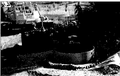
Bild 1: Offener Tandemschacht mit Bewetterung
