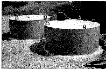
Bild 2: Arbeitstägliche Abdeckung und Absaugung der Tandemschächte.
